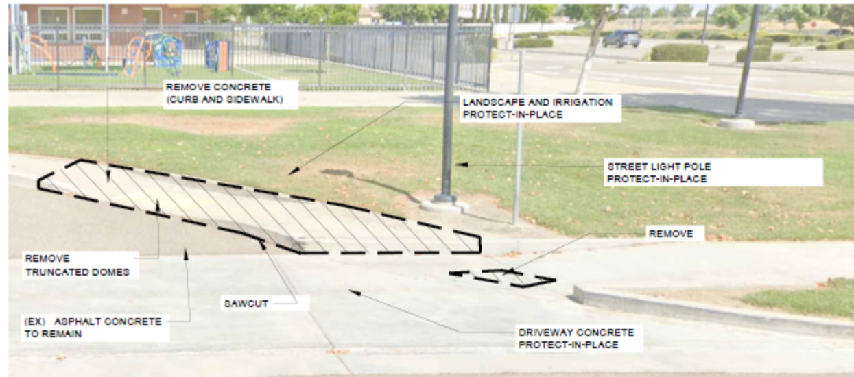
GOLDEN SPIKE TRAIL - SOUTHERLY RAMP DEMOLITION (N.T.S.)
